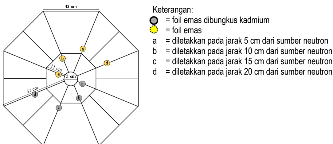
Gambar 1. Ilustrasi Rangka Aluminium Segi Delapan (Jaring Laba-Laba).
