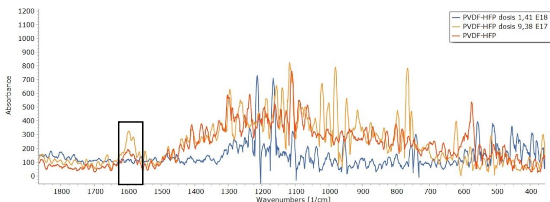
Gambar 11. Spektrum FTIR lapisan tipis PVDF-HFP tanpa implantasi ion, PVDF-HFP dengan dosis implantasi 9,38 \times 10^{17} \text{ ion/cm}^2 dan PVDF-HFP dengan dosis implantasi 1,41 \times 10^{18} \text{ ion/cm}^2 pada bilangan gelombang 1800-400 \text{cm}^{-1} .
