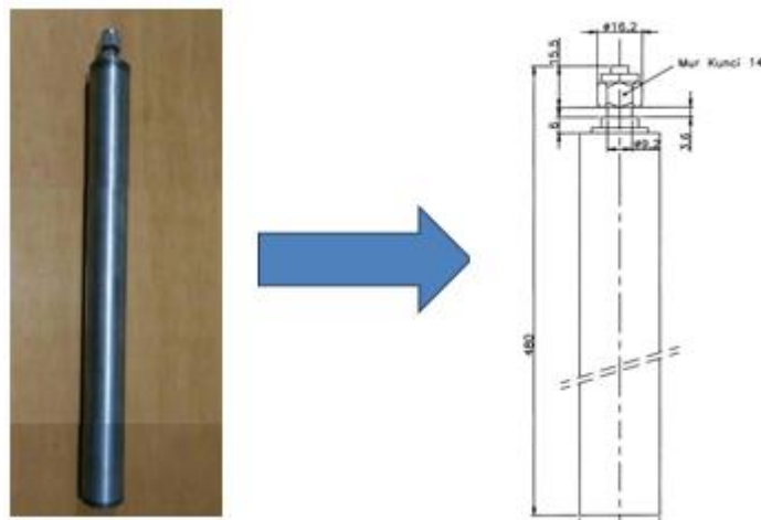
Gambar 3. Tabung kapsul target LEU.
