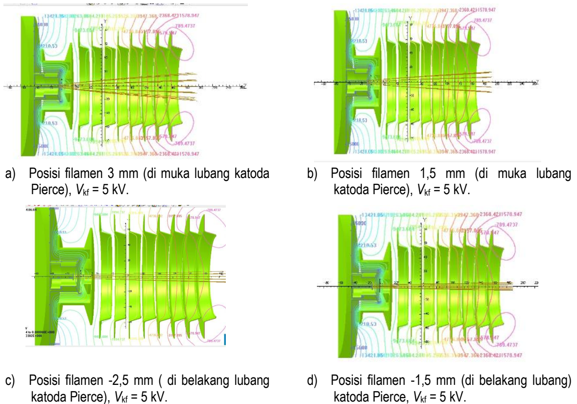
Gambar 5. Pengaruh posisi filamen terhadap lintasan berkas elektron keluar dari SE.
