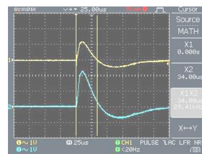
Gambar 6d. Lebar pulsa spot plasma sistem DUET pada permukaan katoda 2 ( \tau = 34 \mu s).
