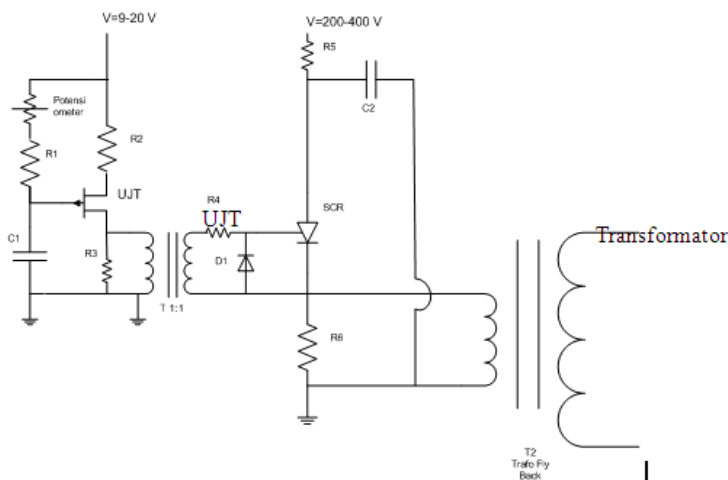
Gambar 2. Rangkaian sistem sumber daya ignitor (IDPS).
