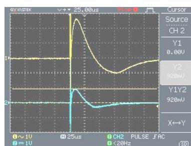
Gambar 4c. Tegangan spot plasma sistem DUET pada permukaan katoda 2 ( V=0,92 V).
