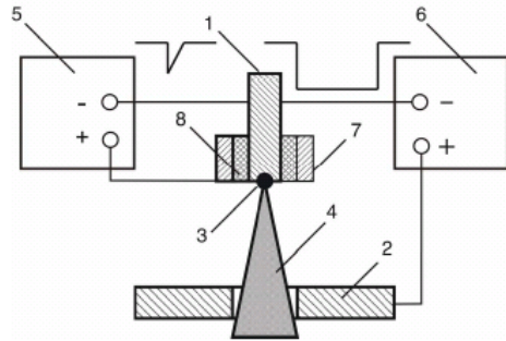
Gambar 1. Diagram sistem elektrode untuk memicu lucutan busur plasma oleh lucutan permukaan pada katode.
