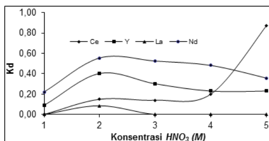
Gambar 5. Hubungan konsentrasi \text{HNO}_3 dengan
