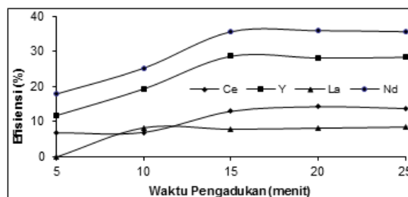
Gambar 4. Hubungan waktu ekstraksi dengan efisiensi ekstraksi
