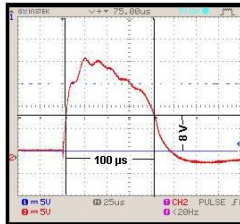
Gambar 4. Pulsa arus I_{ADPS} ( \tau = 100 \mu s , V_t = 8 volt) pada saat P_{Ar} = 8,4 \times 10^{-4} mbar.
