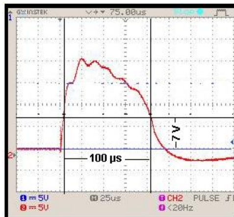
Gambar 6. Pulsa arus I_{ADPS} ( \tau = 100 \mu s , V_t = 8 volt) pada saat P_{Ar} = 24 \times 10^{-4} mbar.
