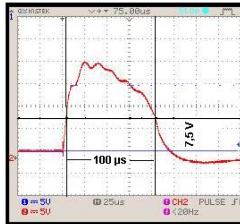
Gambar 5. Pulsa arus I_{ADPS} ( \tau = 100 \mu s , V_t = 8 volt) pada saat P_{Ar} = 14 \times 10^{-4} mbar.
