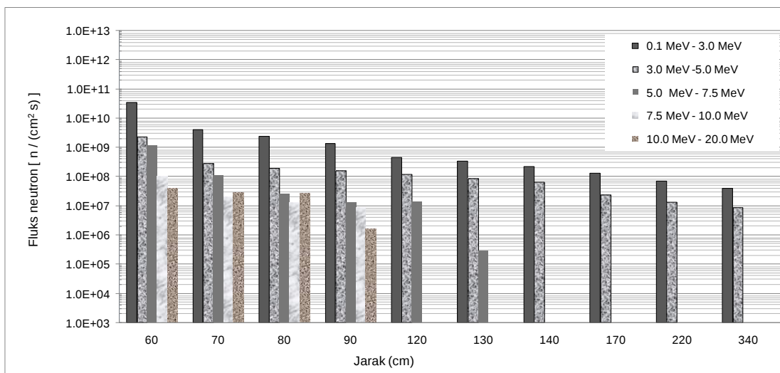
Gambar 7. Karakteristik fluks neutron cepat pada BP2.
