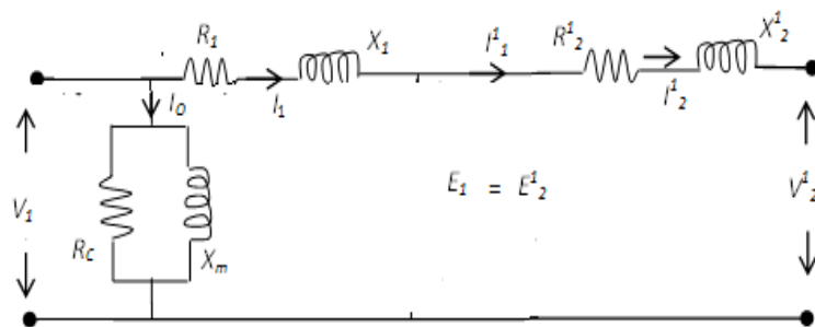
Gambar 3. Rangkaian ekivalen trafo, lilitan sekunder dipindahkan ke sisi primer dan arus tanpa beban diabaikan terhadap arus beban penuh.
