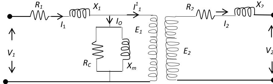
Gambar 2. Rangkaian ekivalen trafo.
