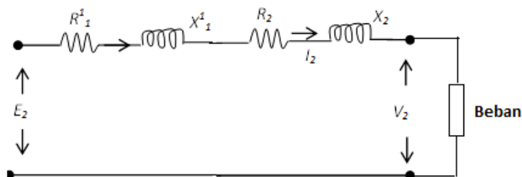
Gambar 4. Rangkaian ekivalen trafo berbeban dilihat di sisi sekunder.
