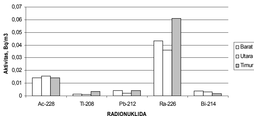
Gambar 8. Hasil identifikasi filter PM 10 dengan spektrometri \gamma
