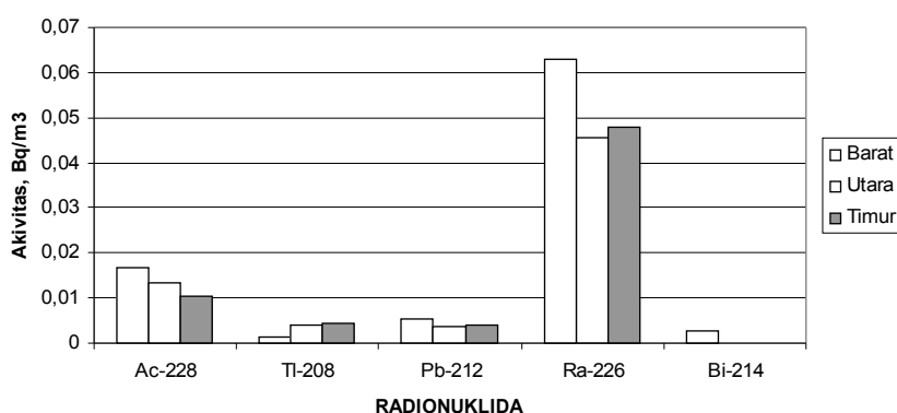
Gambar 7. Hasil identifikasi filter PM 2,5 dengan spektrometri \gamma
