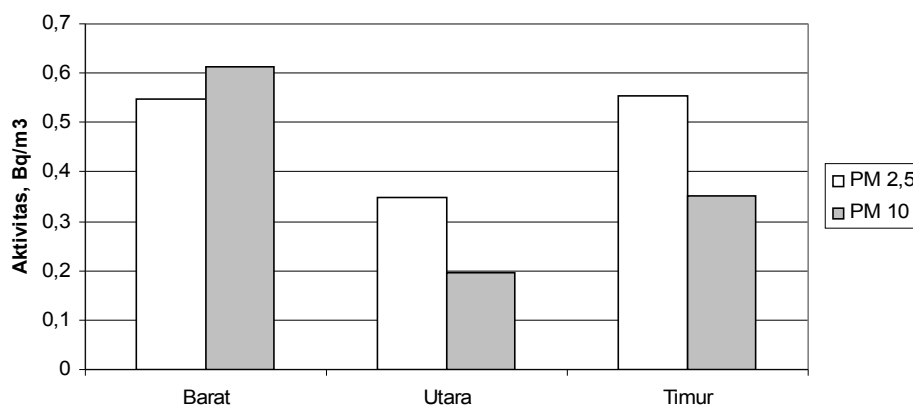
Gambar 9. Hasil identifikasi filter PM 10 dengan spektrometri \gamma
