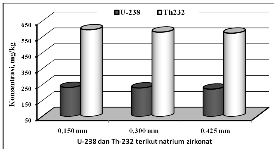
Gambar 2. Histogram U-238 dan Th-232 terikut dalam natrium zirkonat ( \text{Na}_2\text{ZrO}_3 ) dengan berbagai ukuran butir leburan pasir zirkon.
