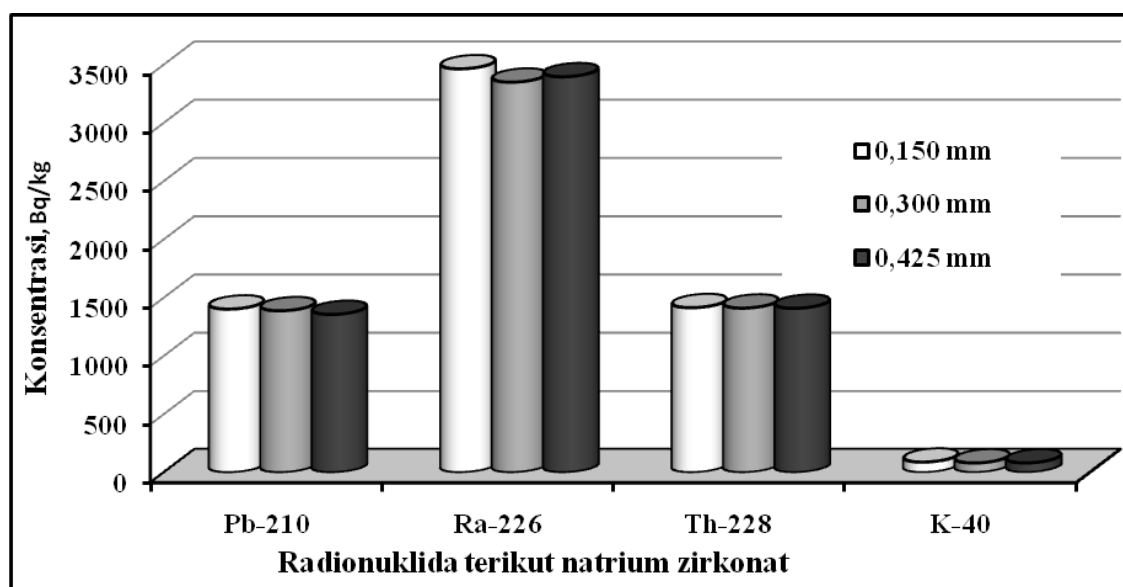
Gambar 1. Histogram TENORM terkandung dalam natrium zirkonat ( \text{Na}_2\text{ZrO}_3 ) dengan berbagai ukuran butir leburan pasir zirkon.
