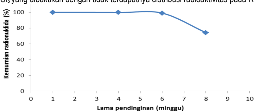
Gambar 4. Pengaruh lama pendinginan terhadap kemurnian radionuklida sediaan radioisotop ^{175}\text{YbCl}_3 hasil iradiasi bahan sasaran ^{174}\text{Yb} diperkaya 98,4%.
