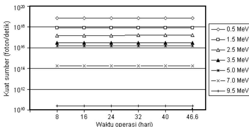
Gambar 6. Grafik distribusi kuat sumber foton hasil peluruhan (foton/detik) dari daerah elemen bakar sebagai fungsi waktu operasi.
