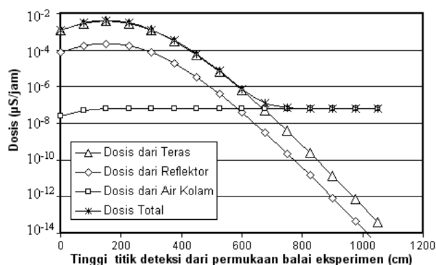
Gambar 10. Dosis pada permukaan dinding di balai eksperimen
