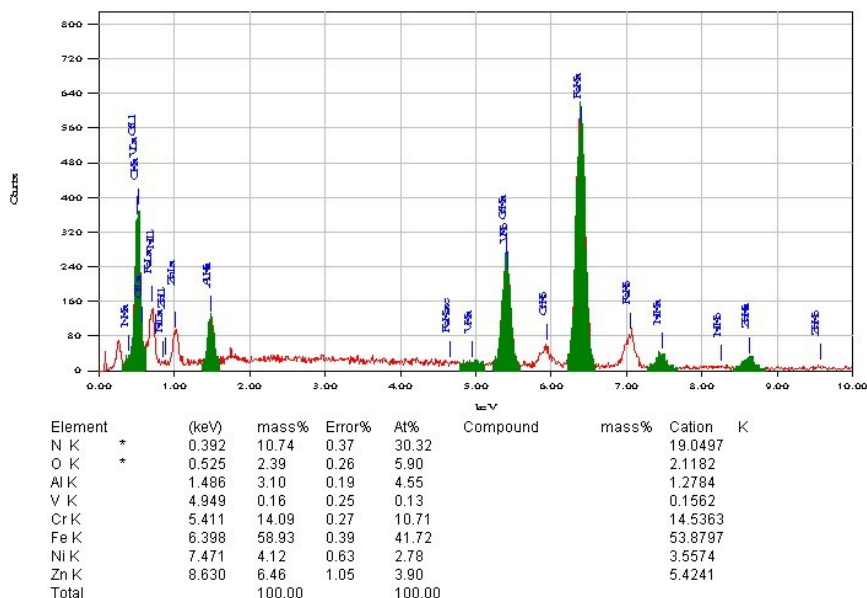
Gambar 7. Hasil Uji EDS material AISI 304 hasil nitridasi plasma pada tekanan 1,8 mbar
