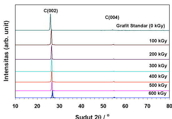
Gambar 1. Pola difraksi sinar-X pelet grafit hasil iradiasi dengan sinar gamma pada dosis (0 - 600 kGy).
