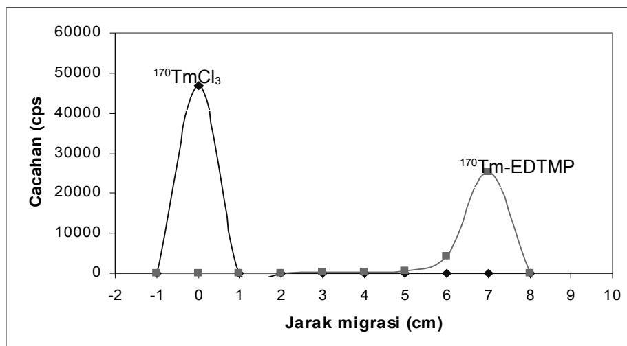
Gambar 1. Hasil kromatografi kertas senyawa kompleks ^{170}\text{Tm-EDTMP} dan senyawa ^{170}\text{TmCl}_3 dengan menggunakan kertas kromatografi Whatman 3 MM sebagai fase diam dan campuran amoniak : metanol : air = 1:10:20 sebagai fase gerak.
