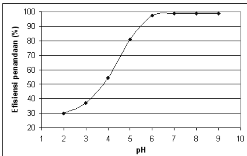
Gambar 5. Pengaruh pH terhadap efisiensi penandaan senyawa ^{170}\text{Tm} -EDTMP.
