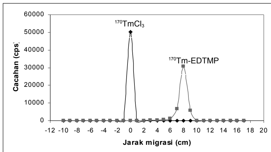
Gambar 2. Hasil elektroforesis kertas senyawa kompleks ^{170}\text{Tm-EDTMP} dan senyawa ^{170}\text{TmCl}_3 .
