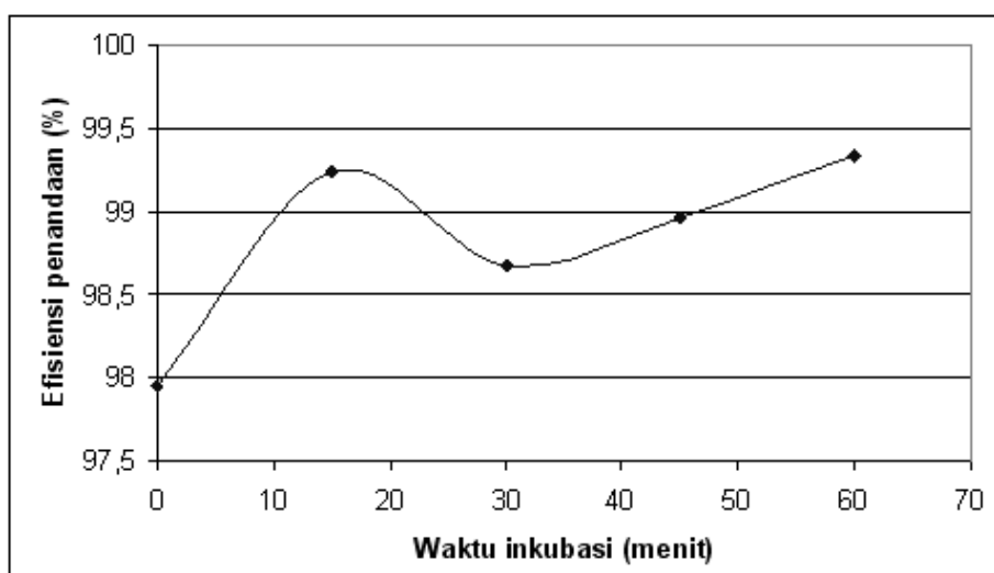
Gambar 6. Pengaruh waktu inkubasi terhadap efisiensi penandaan senyawa ^{170}\text{Tm} -EDTMP.
