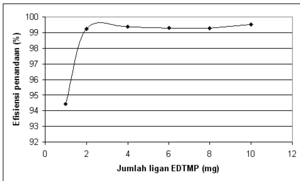
Gambar 4. Pengaruh jumlah ligan terhadap efisiensi penandaan senyawa ^{170}\text{Tm-EDTMP} . Keterangan : pH = 7, t_{\text{inkubasi}} = 30 menit pada temperatur kamar,
