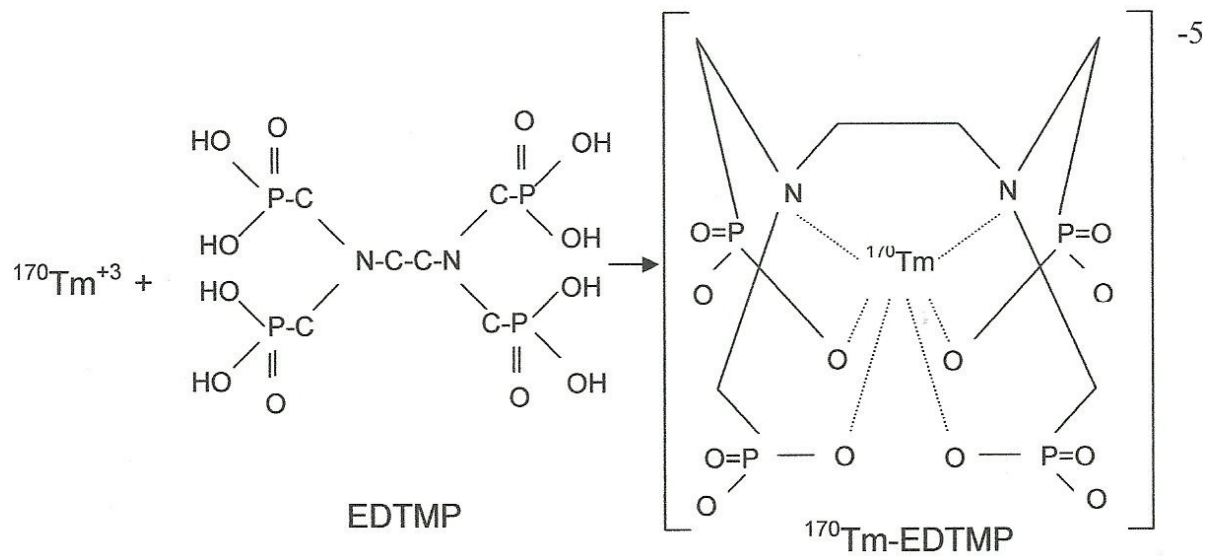
Gambar 3. Struktur kimia senyawa kompleks ^{170}\text{Tm-EDTMP}
