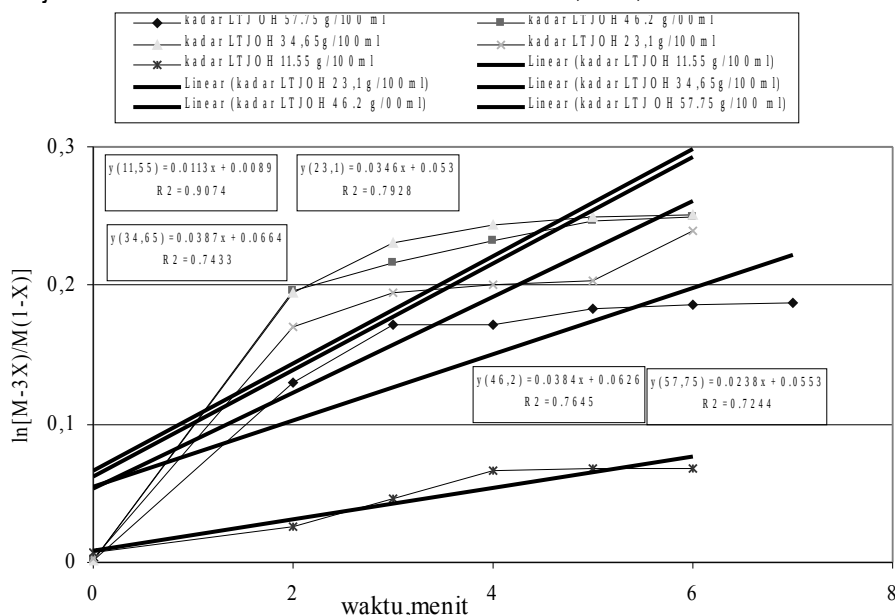
Gambar 11. Grafik hubungan waktu dengan \ln(M-3X)/M(1-X) pada berbagai kadar LTJ hidroksida untuk menghitung harga k jika reaksi orde 2.
