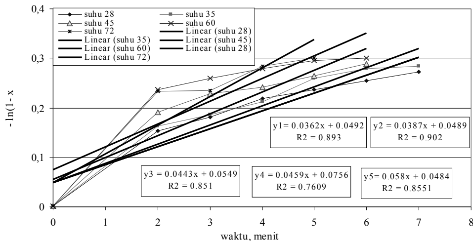
Gambar 3. Grafik hubungan waktu dengan -\ln(1-x) pada berbagai suhu (°C) jika reaksi orde 1.
