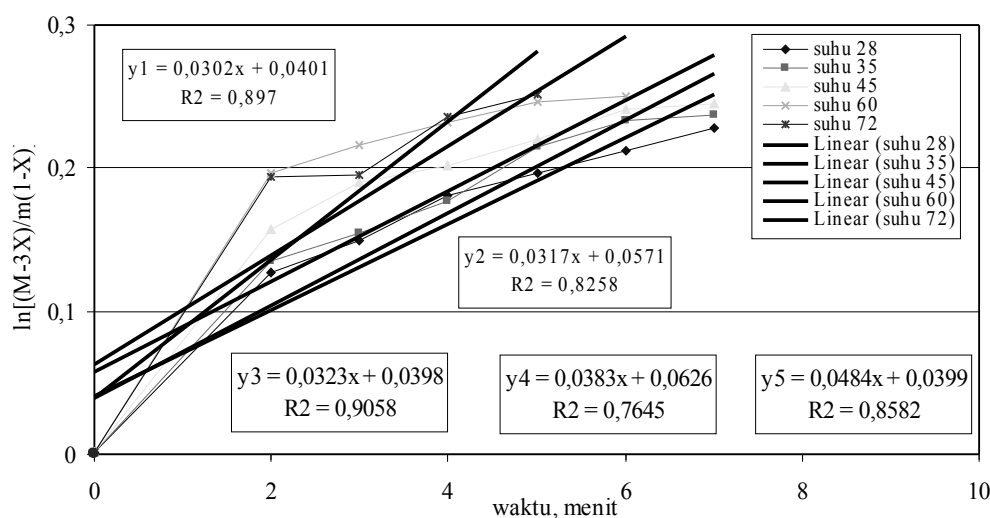
Gambar 5. Grafik hubungan waktu dengan \ln [(M-3X)/M(1-X)] pada berbagai suhu ( ^{\circ}\text{C} ) untuk menghitung harga k untuk reaksi orde 2 bimolekuler.
