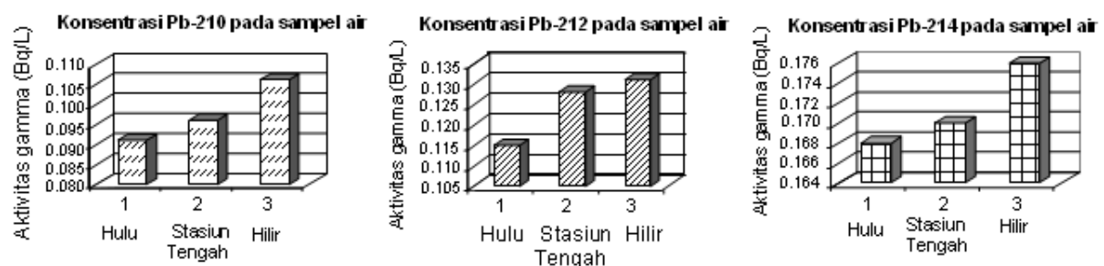
Gambar 4. Aktivitas ^{210}\text{Pb} , ^{212}\text{Pb} dan ^{214}\text{Pb} pada sampel air.
