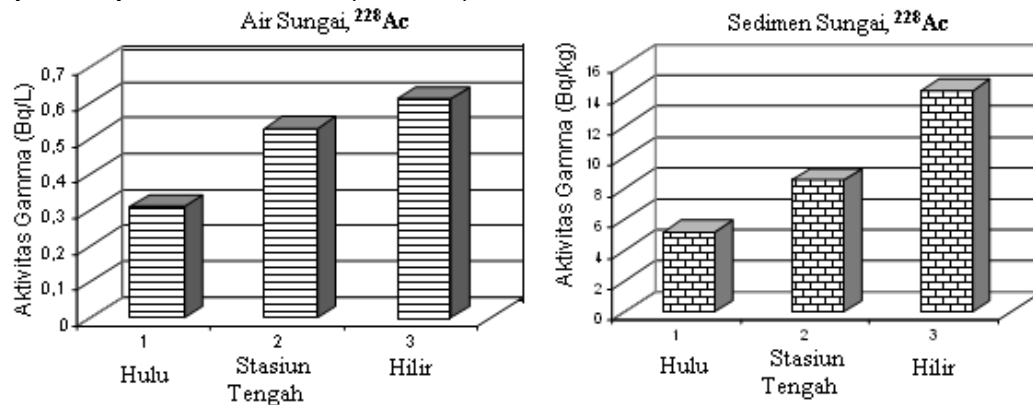
Gambar 8. Aktivitas ^{228}\text{Ac} pada sampel air dan sedimen
