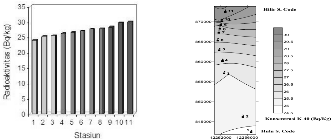
Gambar 11. Diagram peningkatan konsentrasi ^{40}\text{K} dan pola penyebarannya untuk Sampel sedimen sungai Code
