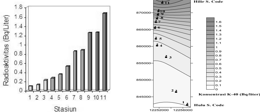
Gambar 10. Diagram peningkatan konsentrasi ^{40}\text{K} dan pola penyebarannya untuk ampel air sungai Code.
