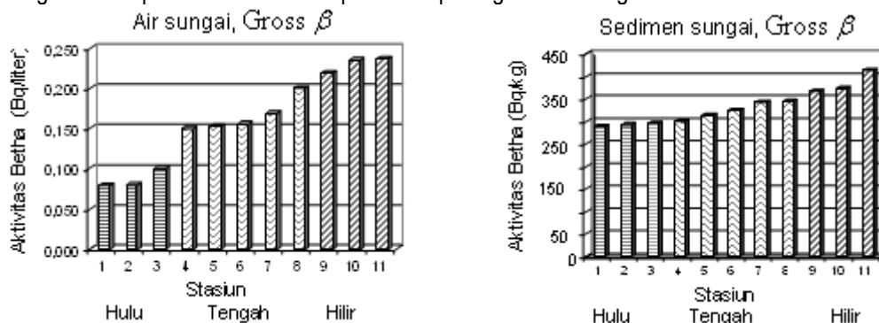
Gambar 3. Pola sebaran gross Beta ( \beta ) pada sampel air dan sedimen dari hulu sampai hilir.
