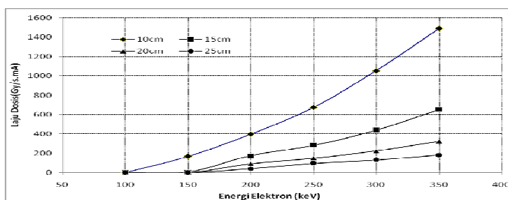
Gambar 5. Laju dosis dosimeter berbasis kalorimeter grafit terhadap energy berkas elektron
