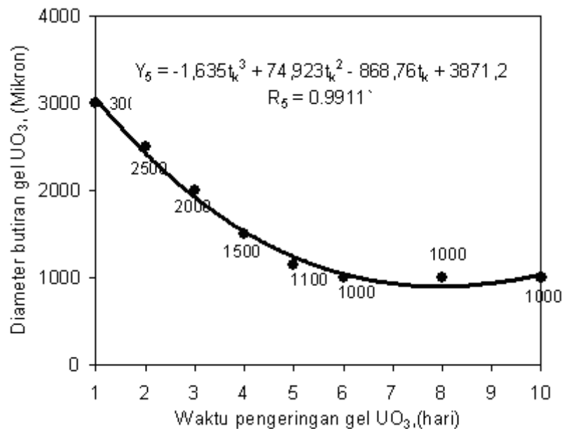
Gambar 6. Pengaruh waktu pengeringan butiran gel \text{UO}_3 pada suhu ruangan terhadap perubahan diameter butiran gel \text{UO}_3 yang diamati dengan mikroskop optik pada pembesaran 50X.
