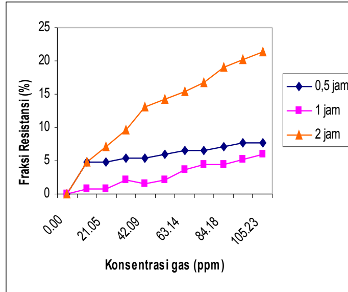
Gambar 4. Sensitivitas sensor terhadap gas CO pada sampel yang dideposisi selama 30 menit, 60 menit dan 120 menit.
