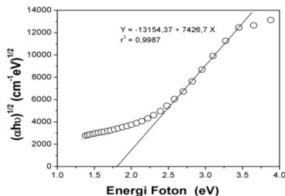
Gambar 6. Grafik koefisien absorpsi optik terhadap energi foton pada panjang gelombang 700 nm untuk lapisan tipis a-Si:H:B pada suhu substrat 200 °C, waktu deposisi 1,5 jam, tekanan gas 1,4 \times 10^{-1} torr dan konsentrasi dopan boron 0,3 %.
