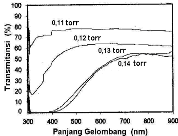
Gambar 5. Spektrum transmitansi optik lapisan tipis a-Si:H:B untuk berbagai tekanan gas pada suhu substrat 200 °C, waktu deposisi 1,5 jam dan konsentrasi dopan boron 0,3 %.
