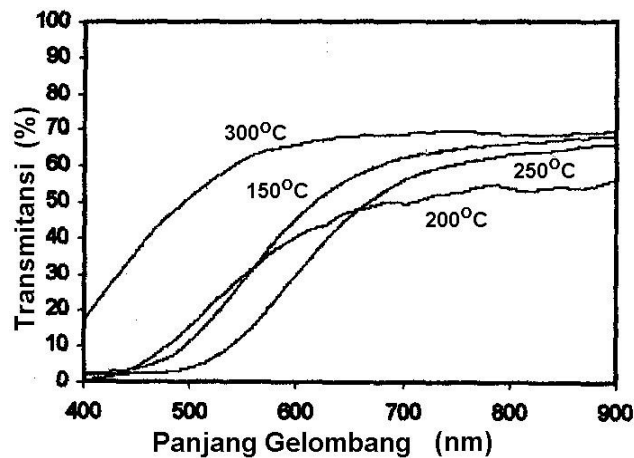
Gambar 3. Spektrum transmitansi optik lapisan tipis a-Si:H:B untuk ber-bagai suhu substrat pada tekanan gas 1,4 \times 10^{-1} torr, waktu deposisi 1,5 jam dan konsentrasi dopan boron 0,3 %.
