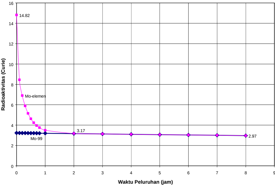
Gambar 6. Perluruhan radioisotop Mo-total dan Mo-99 dalam larutan U-nitrat
