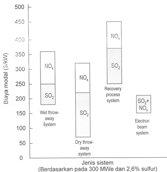
Gambar 4. Biaya modal untuk pengolahan \text{SO}_2 dan \text{NO}_x dalam gas buang ($/kW).
