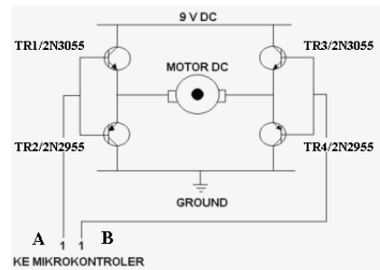
Gambar 4. Susunan jembatan-H ( H-Bridge ) sebagai driver motor DC
