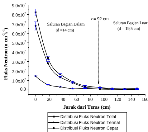
Gambar 8. Kurva Distribusi Fluks Neutron di Saluran Tembus Radial
