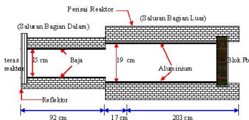
Gambar 2. Saluran Tembus Radial
