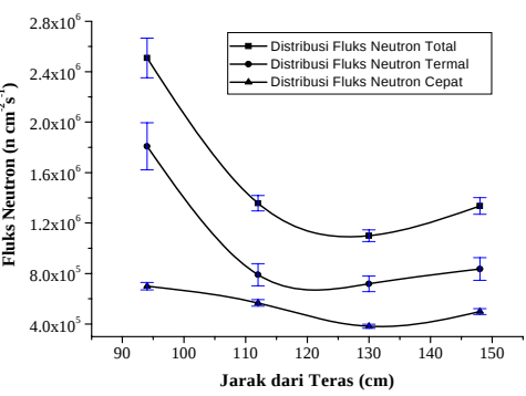
Gambar 7. Kurva Distribusi Fluks Neutron Saluran Tembus Radial Bagian Luar
