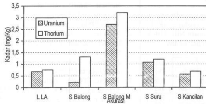
Gambar 1. Histrogram kadar U dan Th terukur berbagai tempat sampling.
