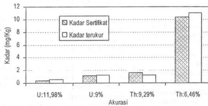
Gambar 2. Histrogram akurasi (%) berbagai kadar untuk U dan Th.
