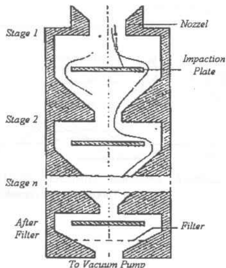
Gambar 4. Impaktor bertingkat
