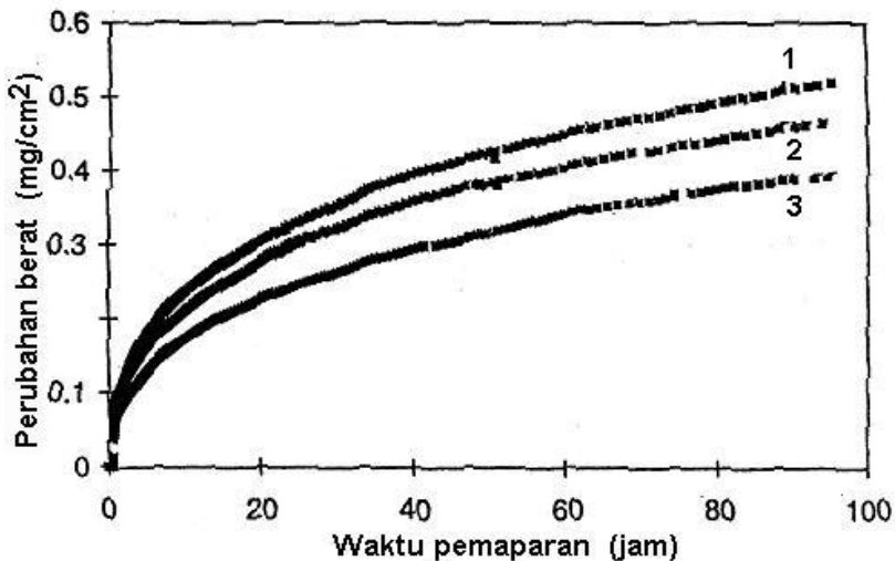
Gambar 1. Hasil uji ketahanan oksidasi suhu tinggi dengan TGA pada suhu 1100^{\circ}\text{C} dalam lingkungan udara yang mengandung oksigen selama 100 jam. Kurve I adalah cuplikan tanpa implantasi (referensi), sedangkan kurve 2 dan 3 masing-masing setelah dilakukan implantasi dengan ion magnesium (Mg) dan yttrium (Y) pada dosis ion 1 \times 10^{18} \text{ ion/cm}^2 dan energi ion 100 \text{ keV} .
