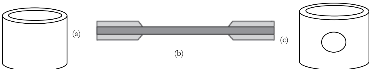
Gambar 2. Bentuk sampel pengujian tekan sejajar serat (a), tarik sejajar serat (b), tarik tegak lurus serat (c) sesuai ISO 22157-2019
