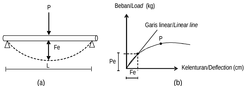
Gambar 1. Pembebanan pada pengujian lentur statik (a) dan grafik hubungan beban dan kelengkungan (b)
