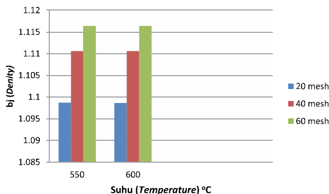
Gambar 4. Bobot jenis bio-oil rumput gelagah pada suhu 550 - 600°C dengan ukuran 20, 40, dan 60 mesh
