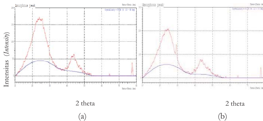
Gambar 7. Difraktogram arang (a) bambu dan (b) jati yang dikarbonisasi suhu 800^{\circ}\text{C}
