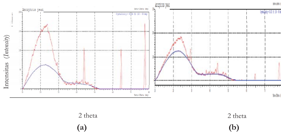
Gambar 6. Difraktogram arang (a) bambu dan (b) jati yang dikarbonisasi suhu 400^{\circ}\text{C}
