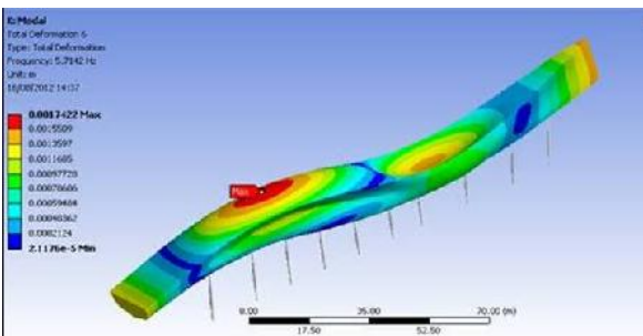
Gambar 8. Mode shape kedua untuk kondisi basah ( wet mode ) dengan koefisien slamming
