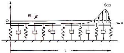
Gambar 1. Model getaran dari lambung kapal
