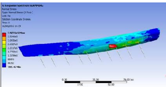
Gambar 9. Respons spektrum kondisi slamming
