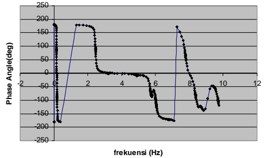
Gambar 11. Sudut Fasa Respons Harmonik kondisi Slamming
