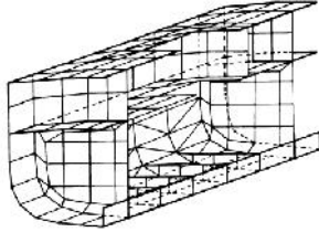
Gambar 3. Penegar - penegar kapal yang didiskritkan oleh elemen hingga
