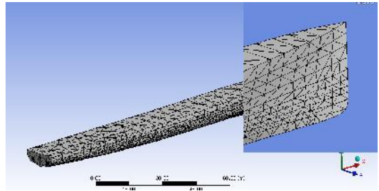
Gambar 5. Diskritisasi dengan triangular elemen badan Kapal Frigate ESC40DV
