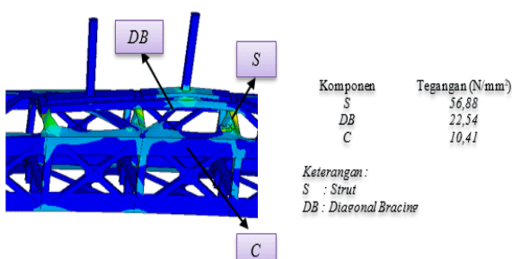
Gambar 16. Nilai tegangan pada komponen area katrol dengan model pondasi diagonal bracing
