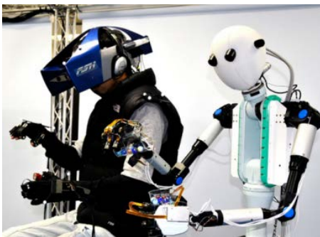
Gambar 12. TELESAR V robot avatar (Sumber : www.infoniac.com )
