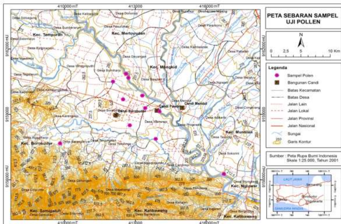
Gambar 6. Peta sebaran sampel pollen di daerah Borobudur dan sekitarnya
