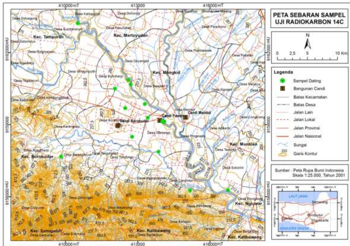
Gambar 8. Sebaran lokasi pengambilan sampel uji radiokarbon ^{14}\text{C} di daerah penelitian
